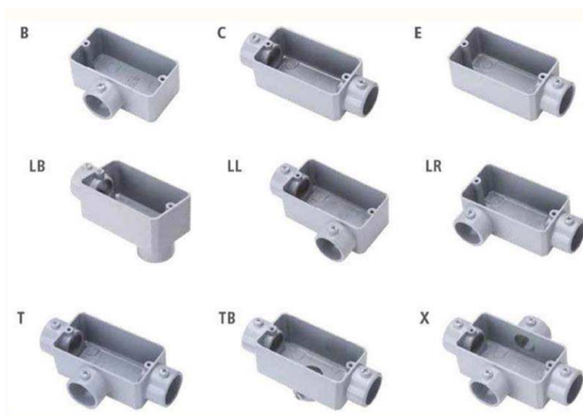
Figura 8 - Referência de modelo de conduteles plásticos
