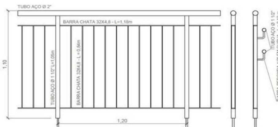
Figura 10 - Layout do Guarda corpo e corrimãos metálicos
